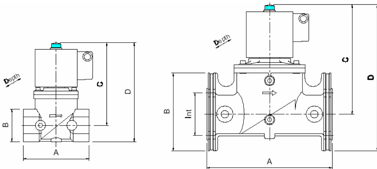
Размеры, мм
